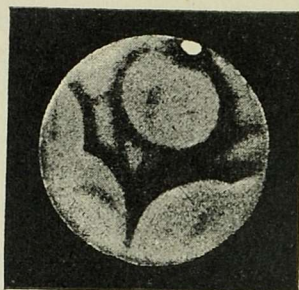
MARS IN 1877 ( Trouvelot ).
