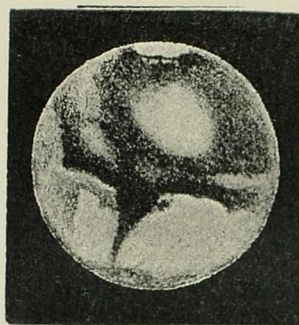
MARS IN 1877 ( N. Green ).
